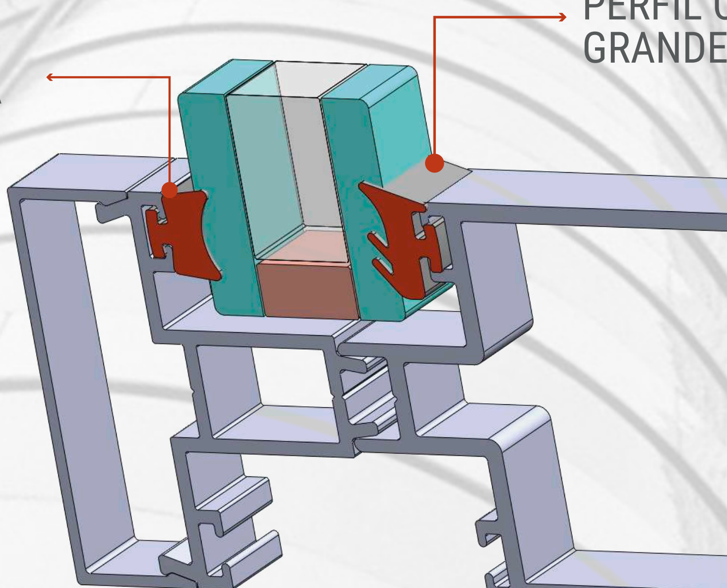
C041389 PERFIL CUÑA ESPACIADORA
