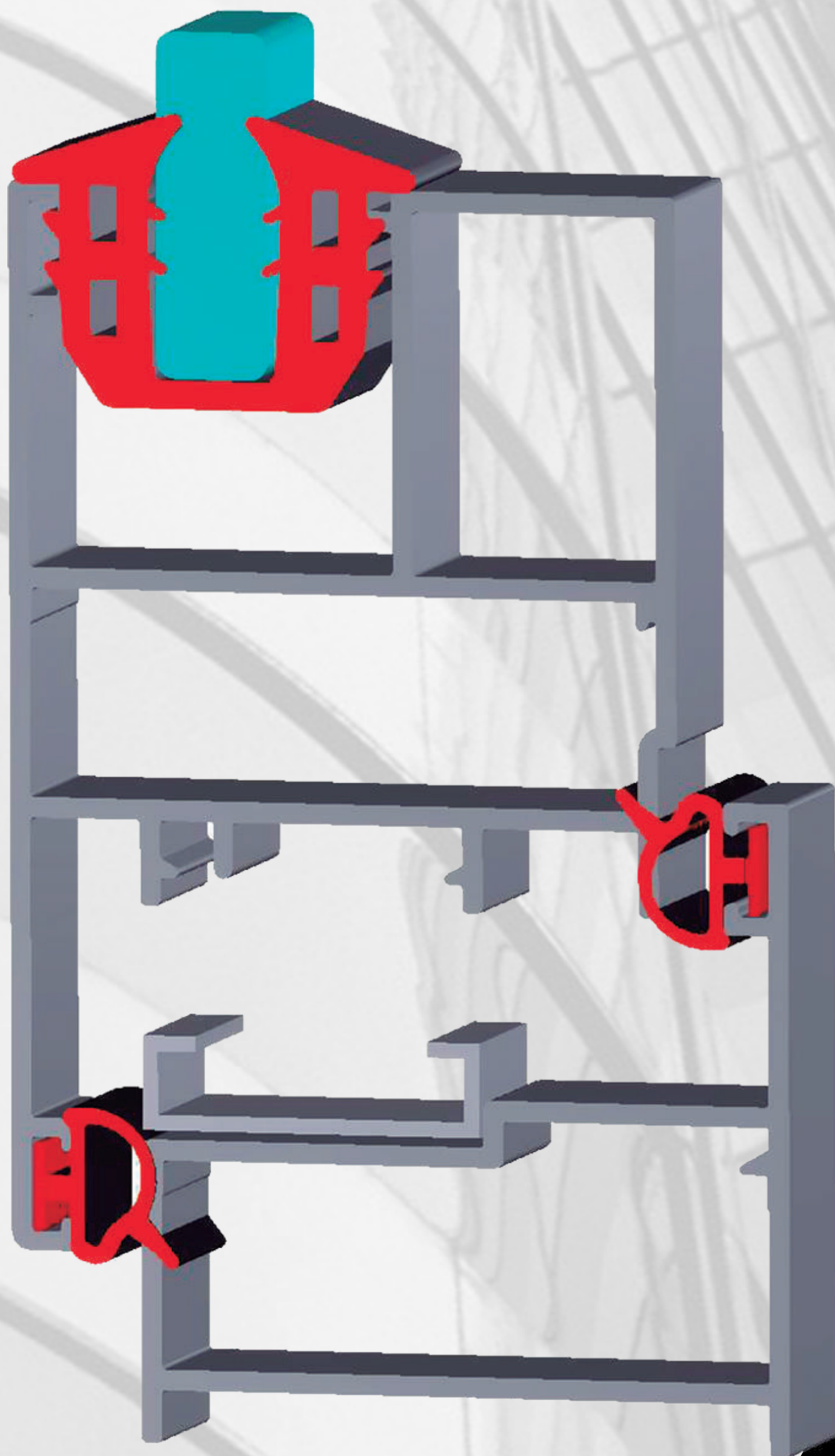
C030674A 17196 Perfil U vidrio de 6 mm SERIE 80
