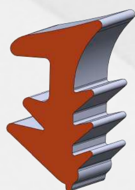
C040215 PERFIL CUÑA MÓVIL
