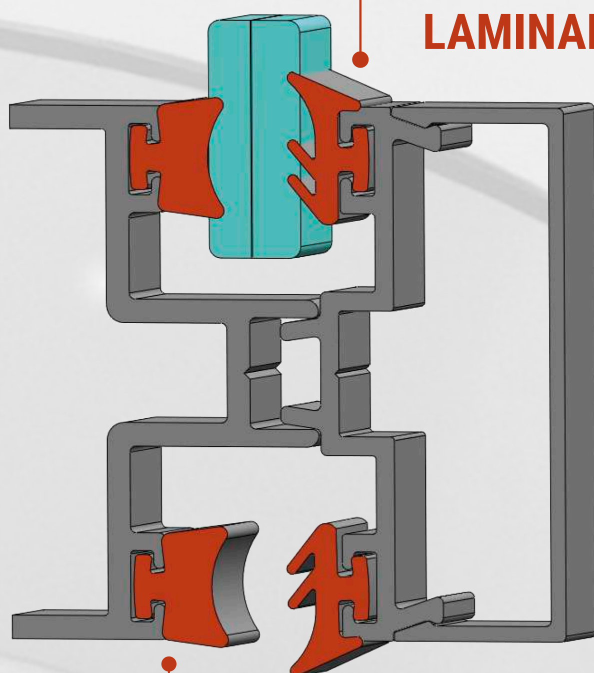
C041389 PERFIL CUÑA ESPACIADORA
